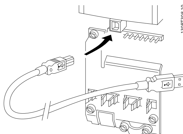
Ilustración 2.25 Conexión USB
