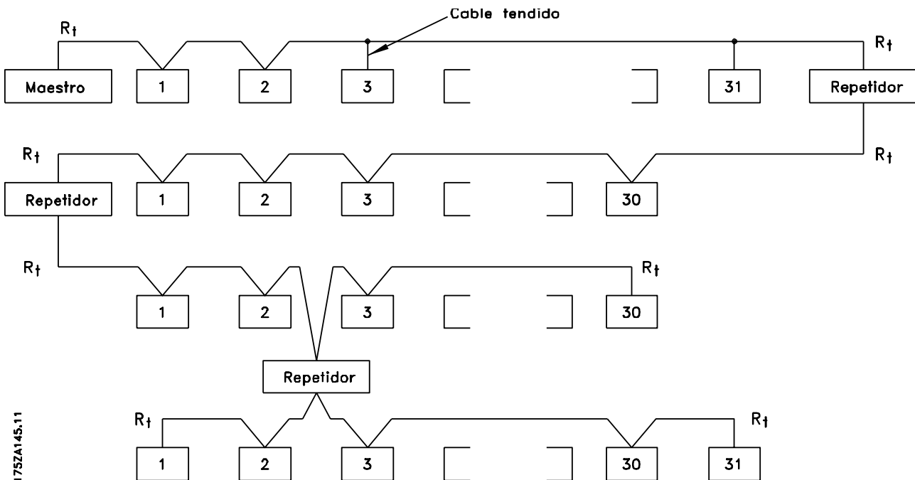
Ilustración 3.40 Interfaz de bus RS485
