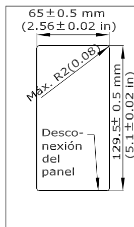
Ilustración 3.37 Dimensiones del kit LCP
