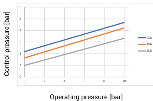
EPDM - Actuator 0KN, 1KN, 2KN
