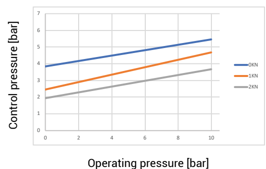
PTFE - Actuator 0KN, 1KN, 2KN
