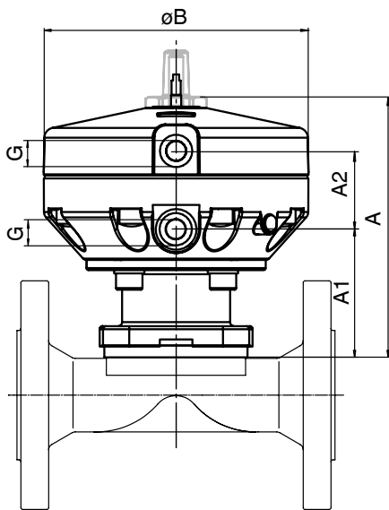
Actuator size 0-2 0KN, 1KN, 2KN
